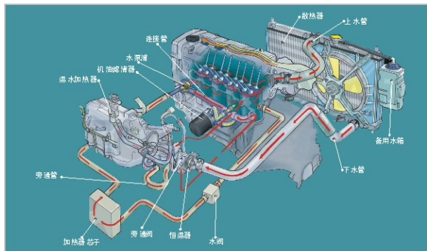
(冷却系统构造)
